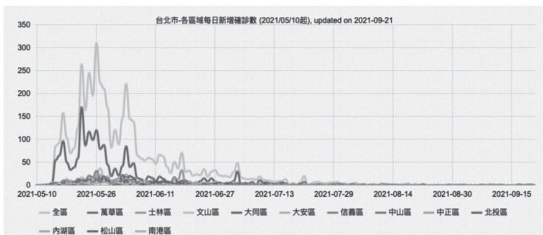
圖 1：臺北市疫情每日統計圖
